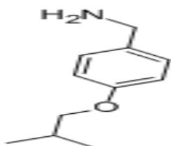
4-(2-METHYLPROPOXY)-BENZENETHANAMINE
